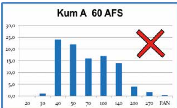
ŞEKİL 1 60 AFS silis kumu (kullanımı uygun değil).
