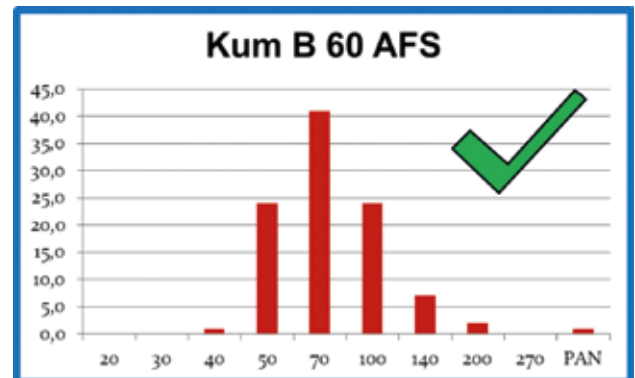
ŞEKİL 2 60 AFS silis kumu (kullanımı uygun).
